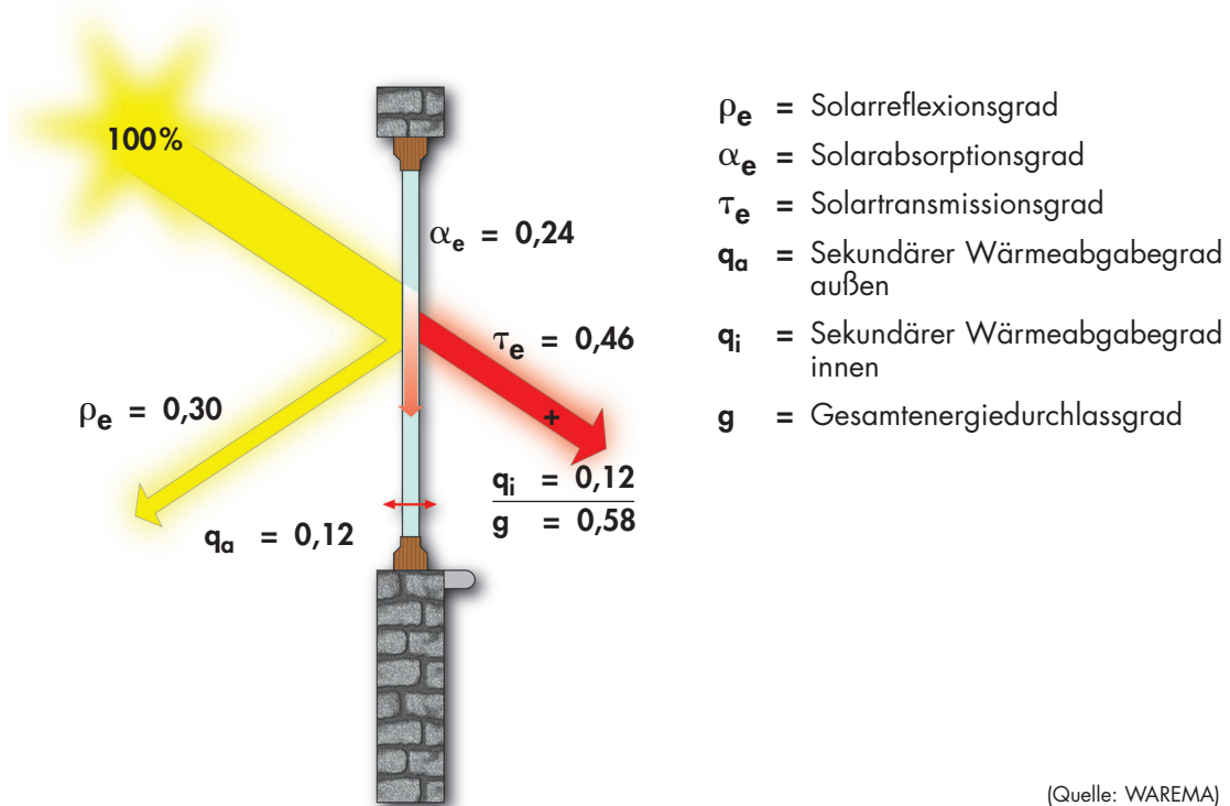
Abb. 2.3-2: Transmission, Reflexion, Absorption an einer Wärmeschutzverglasung
