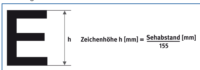
Abbildung 16: Minimale Zeichenhöhe
